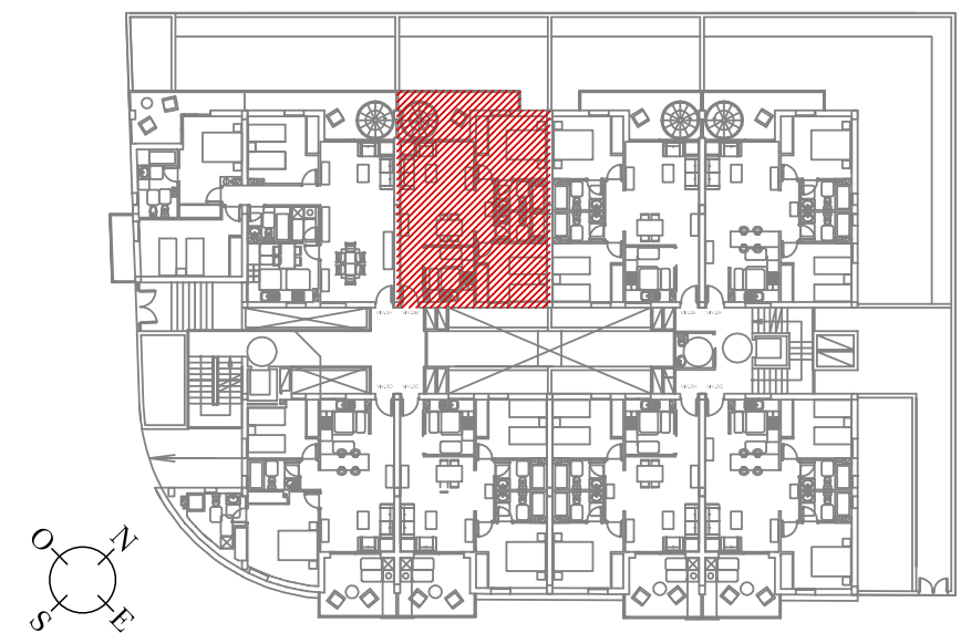
PLANTA SEGUNDA
