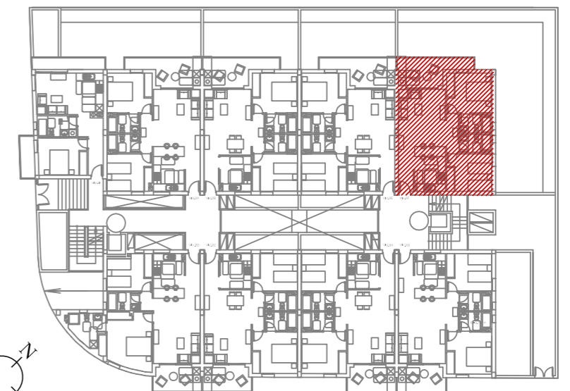
PLANTA PRIMERA
