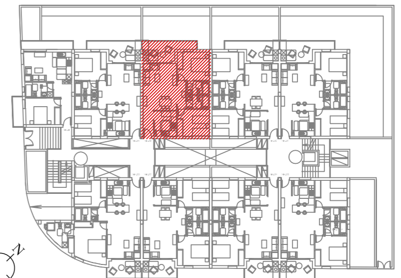
PLANTA PRIMERA
